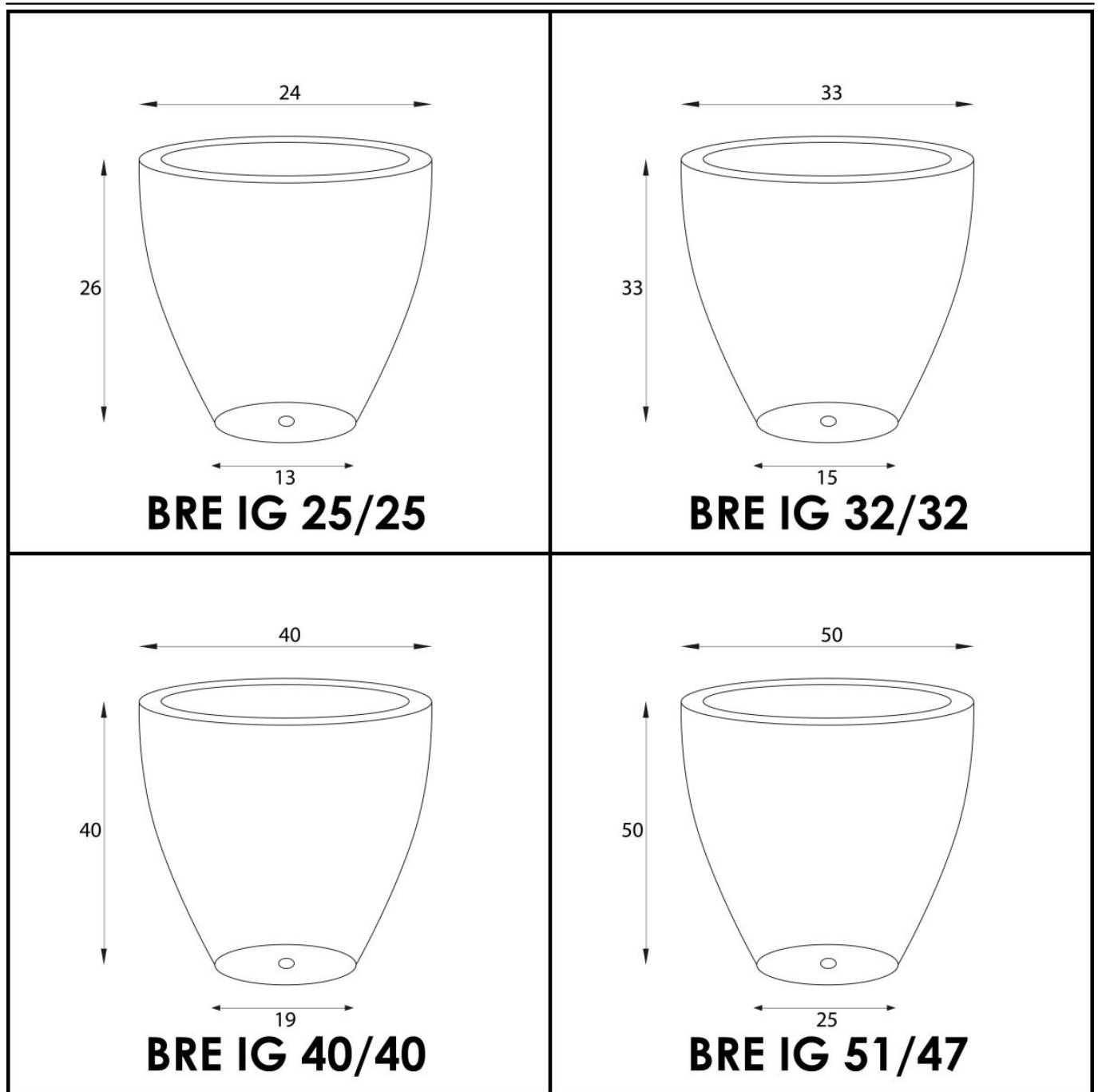
Wymiary zestawu czterech doniczek ceramicznych BRE IG
