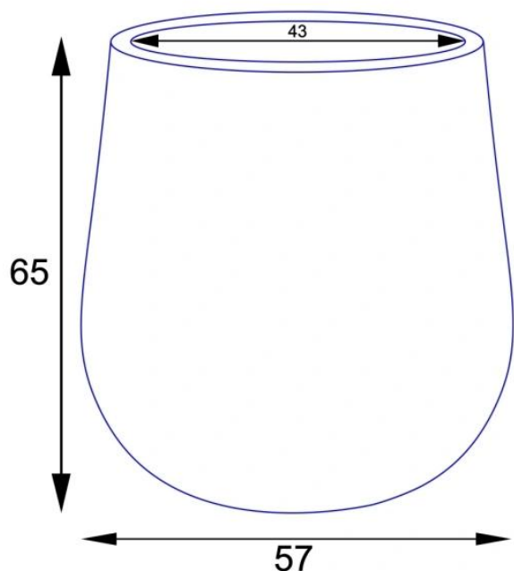
Wymiary donicy SQ65 szary beton - wersja bez wewnętrznego wkładu
