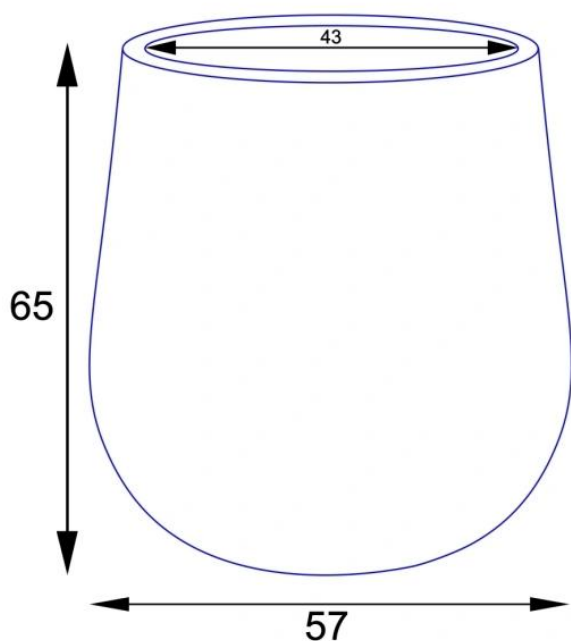
Wymiary donicy SQ65 grafitowy beton - wersja bez wewnętrznego wkładu
