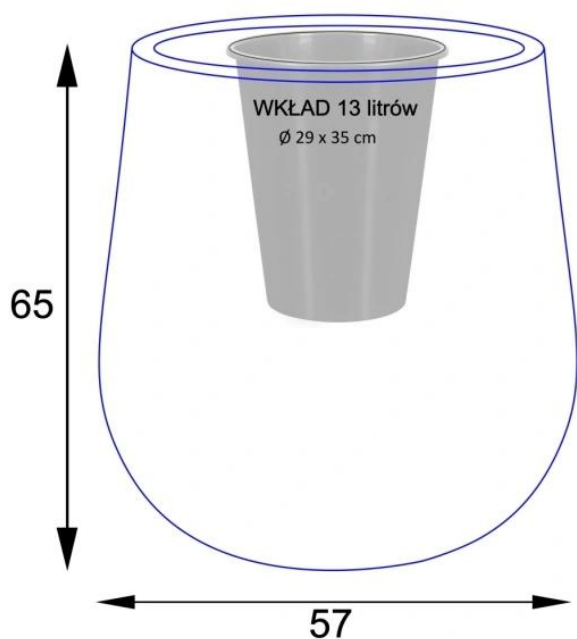
Wymiary donicy SQ65 grafitowy beton - wersja z wewnętrznym wkładem
