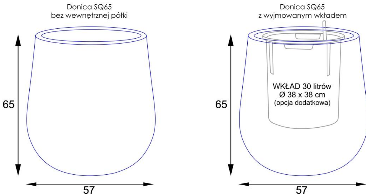
Porównanie opcji donicy SQ65: bez wkładu i z wewnętrznym wkładem
