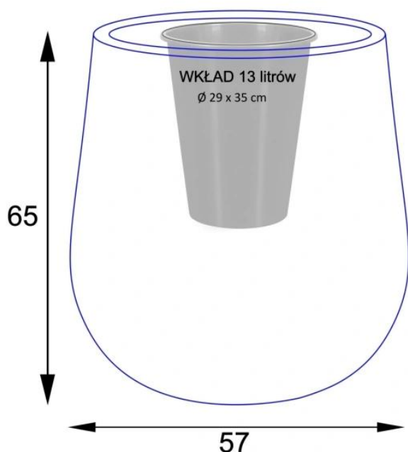
Wymiary donicy SQ65 antracyt mat - wersja z wewnętrznym wkładem
