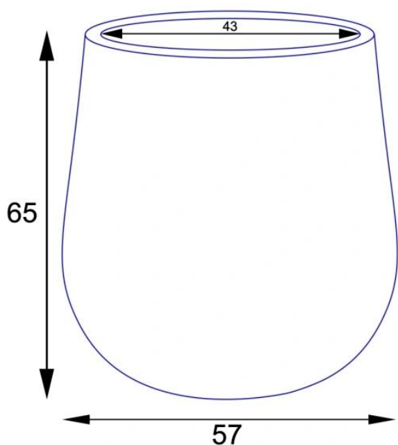
Wymiary donicy SQ65 antracyt mat - wersja bez wewnętrznego wkładu
