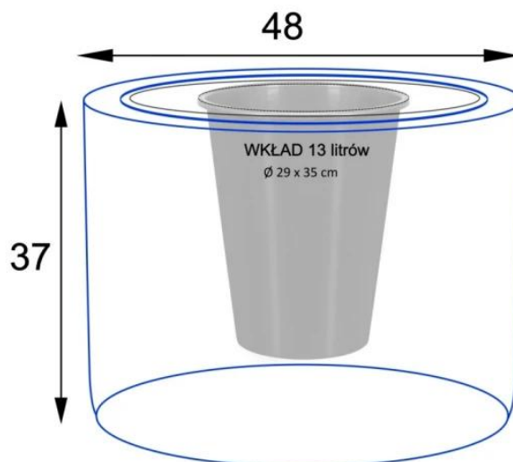
Doniczka LEO37 grafitowy beton - wersja z wewnętrznym wkładem
