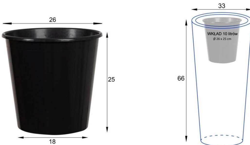
Wymiary wewnętrznego wkładu | Wymiary donicy D208D/BPD
